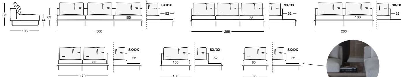
Centrali / Central / Центральные секции
