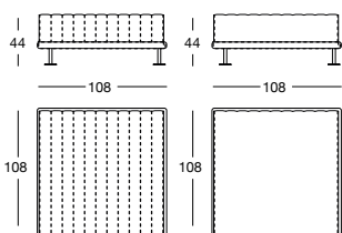
Pouf / Ottoman / Пуф
