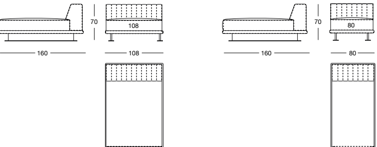
Dormeuse senza braccioli / chaise longue without armrests / шезлонг без подлокотников
