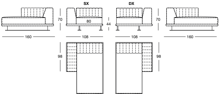
Angolo / Corner / Угловой элемент
