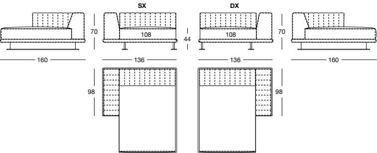
Dormeuse con braccioli / chaise longue with armrests / шезлонг с подлокотниками
