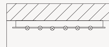
Altezza - Height MIN 7 cm - 2.75"
