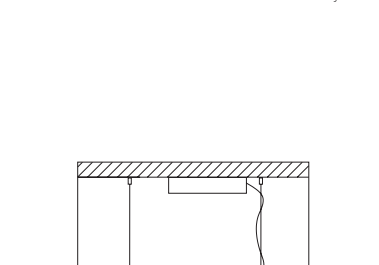
F Altezza - Height MIN 24 cm - 9.44" Aggancio con rosone, tiranti e tasselli a soffitto; altezza regolabile (F) - Hook with ceiling cup, metal cables and ceiling cable gripper; adjustable height (F) * rosone scatola rettangolare L15 W7 H3,5 cm - rectangular metal box L15 W7 H3,5 cm
