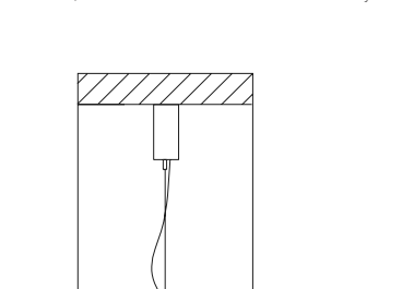
A Altezza - Height MIN 30 cm - 11.8" Aggancio con rosone o scatola in metallo e tirante in metallo; altezza regolabile (A) - Hook with ceiling cup or metal box and metal cable; adjustable height (A) * rosone cilindrico Ø7 H16 cm - cylindric metal box Ø7 H16 cm
