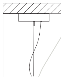
Altezza - Height MIN 18 cm - 7.08"
